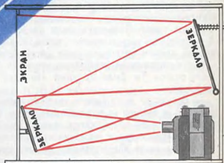
СХЕМА РАСПОЛОЖЕНИЯ ЗЕРКАЛ, И ХОД ЛУЧЕЙ
