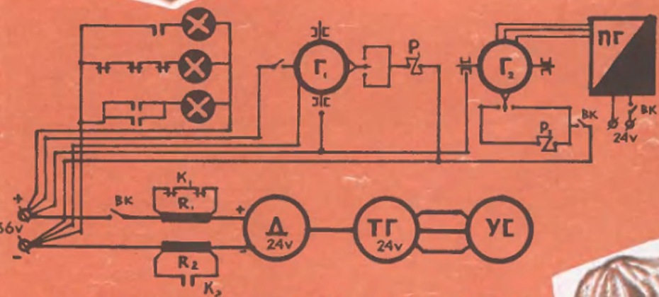
ЭЛЕКТРИЧЕСКАЯ СХЕМА «АВТОМАШИННИСТА»
