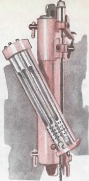
Термометр для измерения температуры морской воды на любой глубине.
